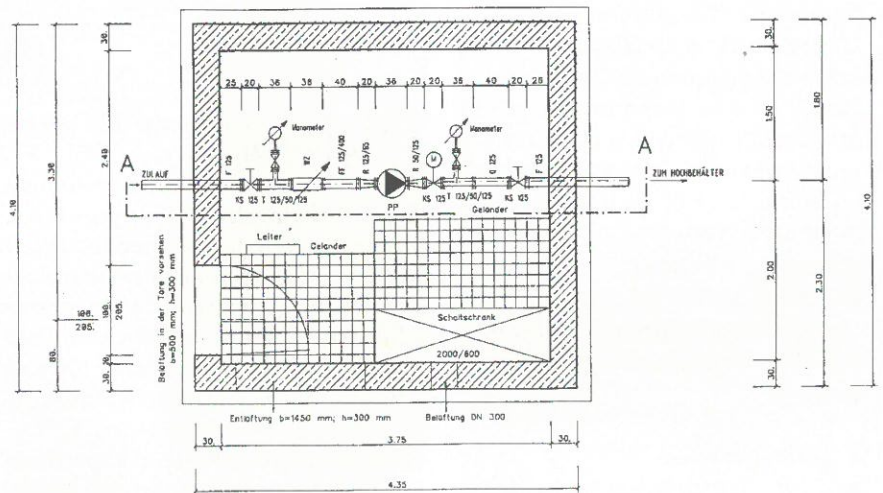
Im Grundriss: Die neue Pumpstation für die Wasserzuleitung aus den Alpeil-Quellen. Zeichnung: Ingenieurbüro Pesjak
